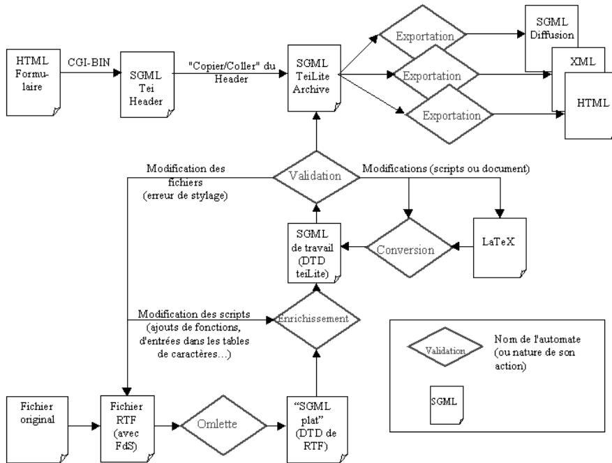
FIG. 2 – Organigramme du processus de production de SGML.
