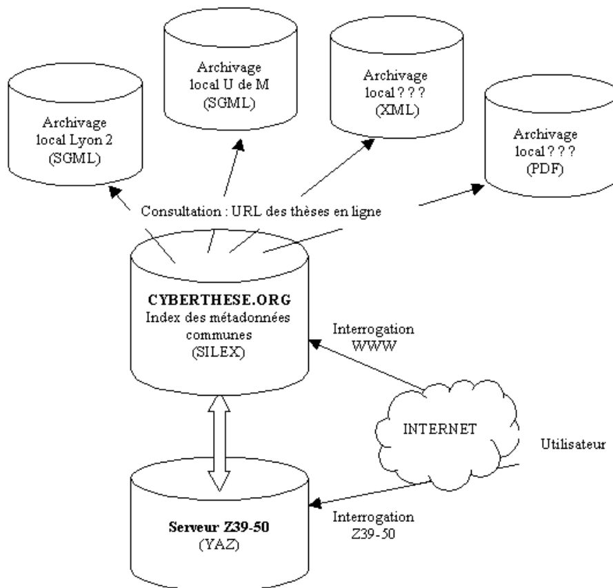
FIG. 3 – Architecture du portail CyberThèses.
