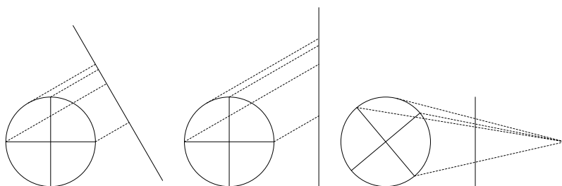
Figure 1. — Projections orthogonale (à gauche), oblique (au milieu) et perspective (à droite).
